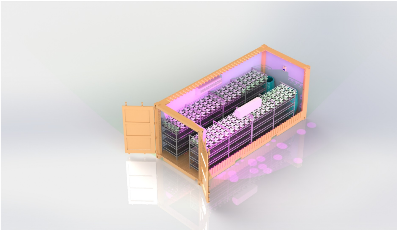
Gambar 1 - Tampak Perspektif
